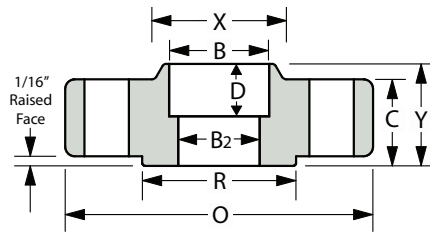
SOCKET WELD (SW)
